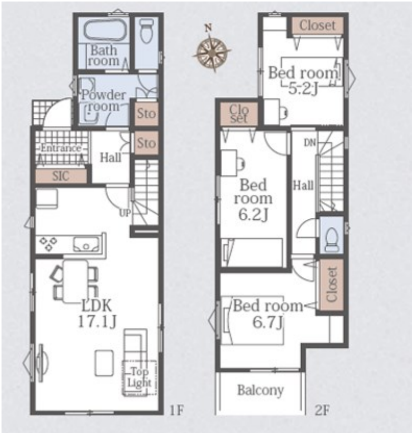
【間取り図】
