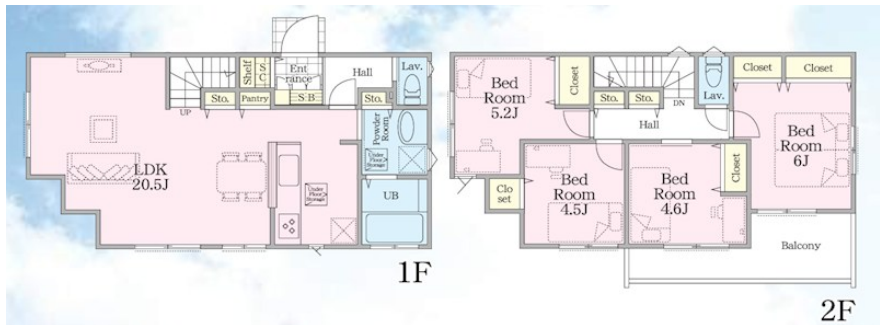
【間取り図】
