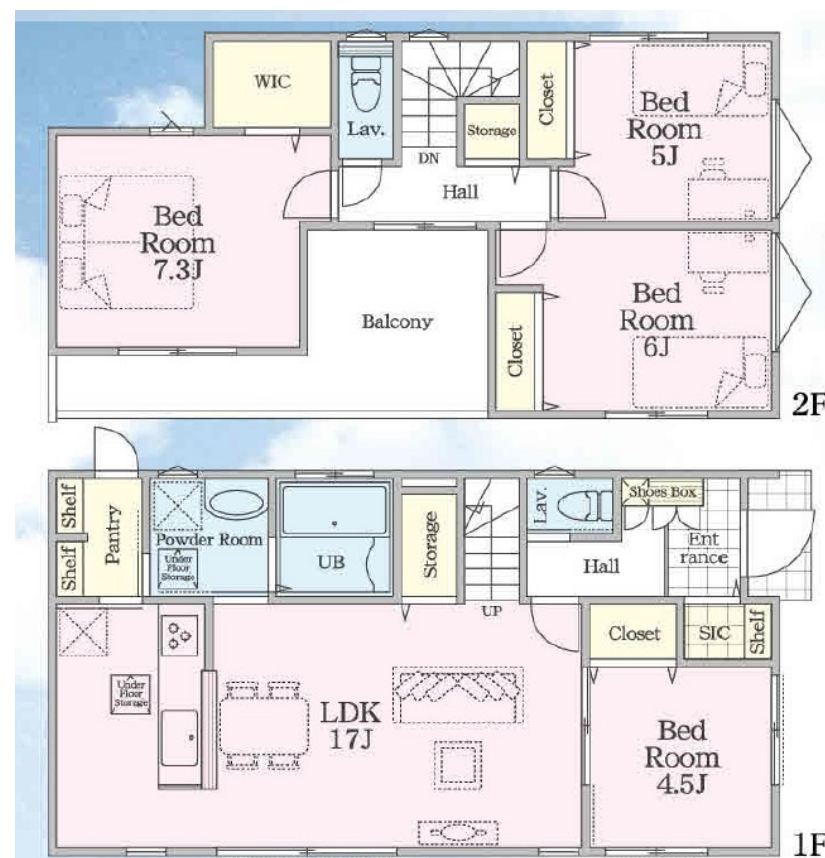
【間取り図】
