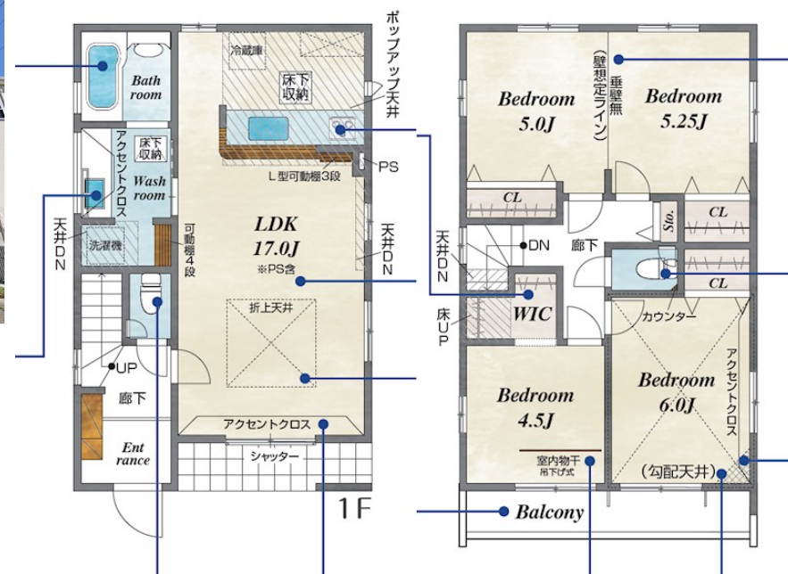
【間取り図】
