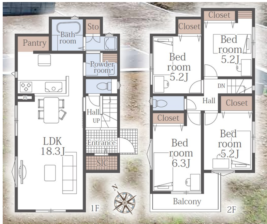
【間取り図】
