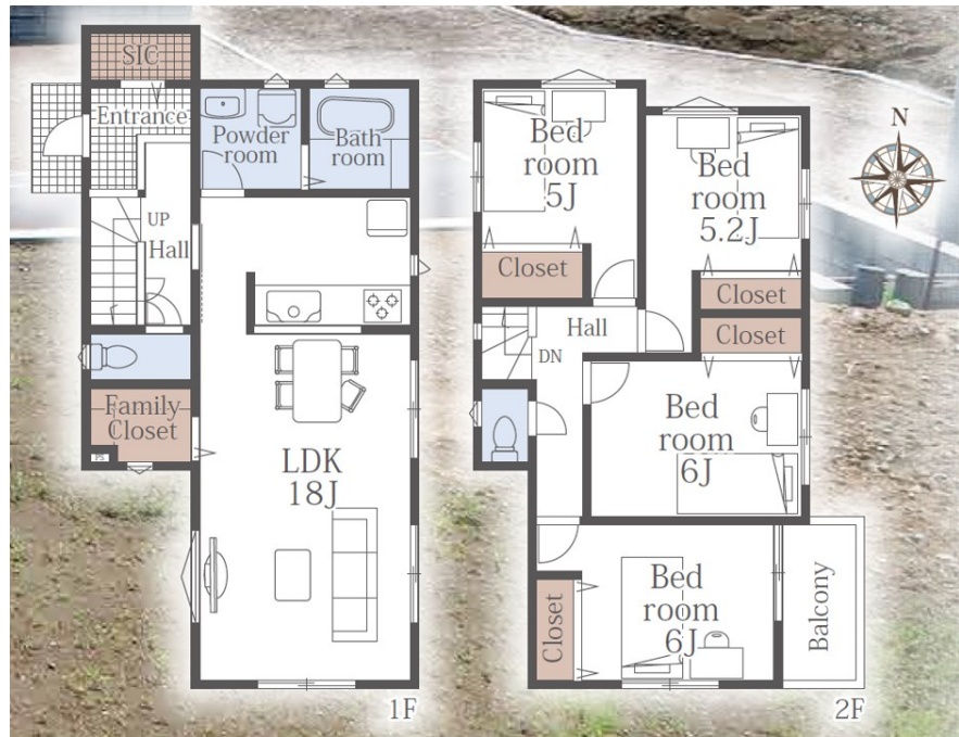
【間取り図】
