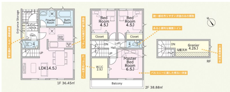
【間取り図】
